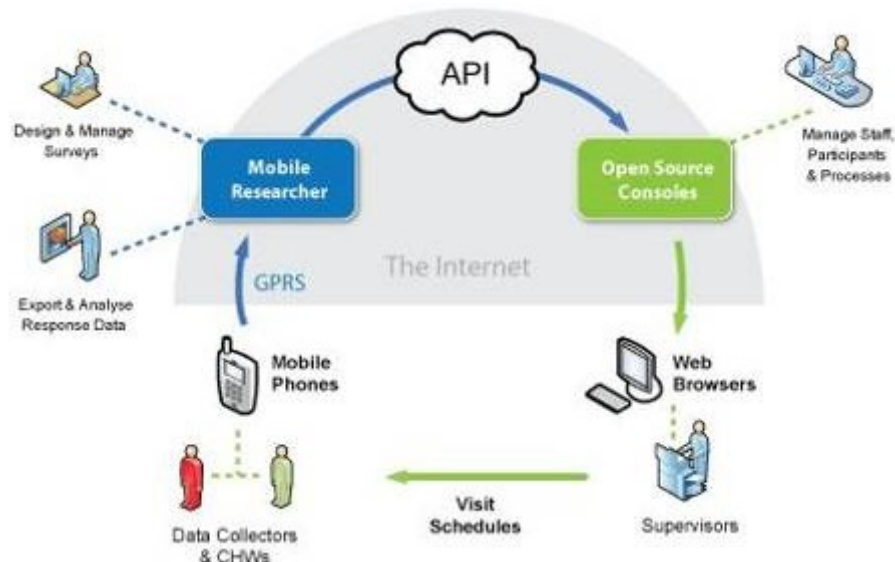
Gambar 1. Konsep API
