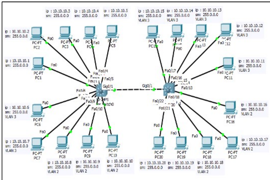
Gambar 6. Desain Vlan pada switch
