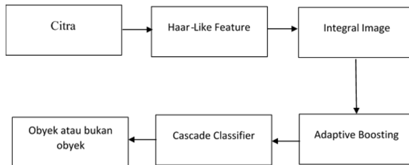
Gambar 1. Skema Proses Deteksi Obyek dengan Metode Viola-Jones.
