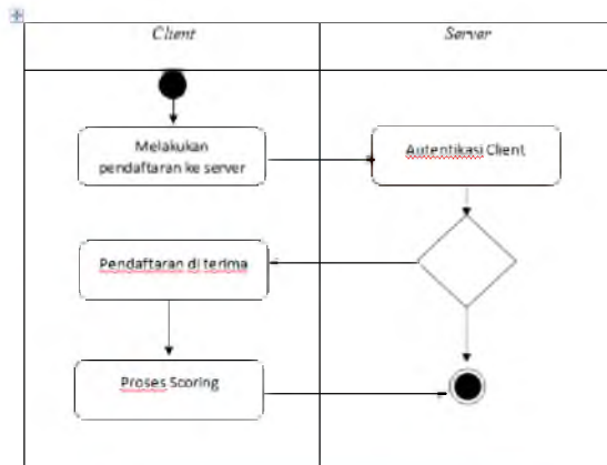
Gambar 2 Activity Diagram keseluruhan sistem
