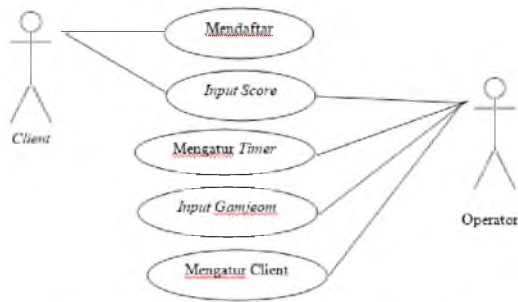
Gambar 1. Use Case Diagram keseluruhan sistem
